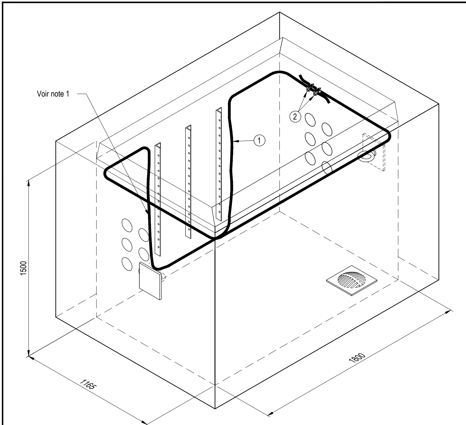
Vue isométrique
